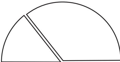
semi-circle
