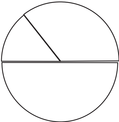
circle
